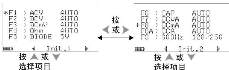
图 4-26 在初始功能页之间导航
