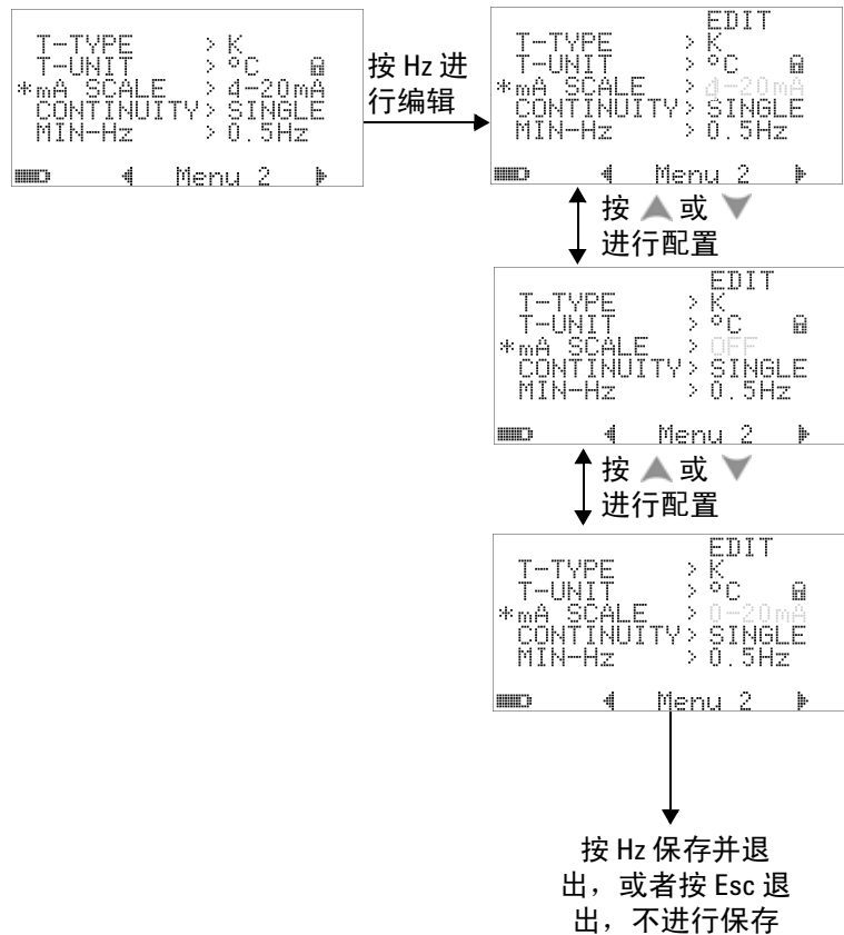
图 4-9 设置百分比刻度读数
