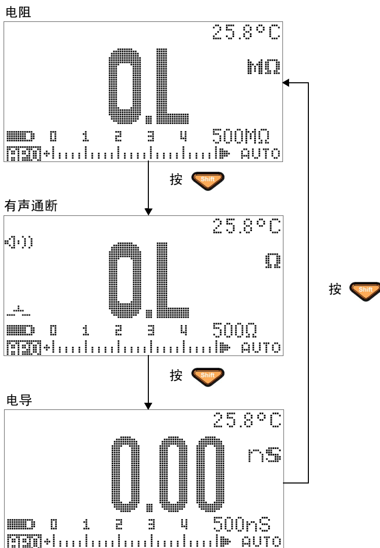
图 2-9 电阻、有声通断和电导测试
