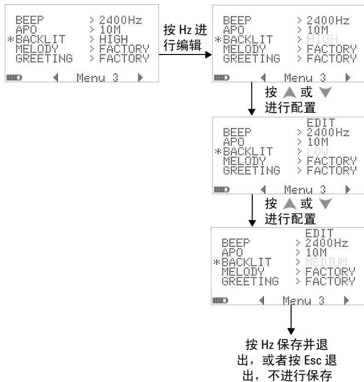
图 4-14 电源打开时的背光灯设置
