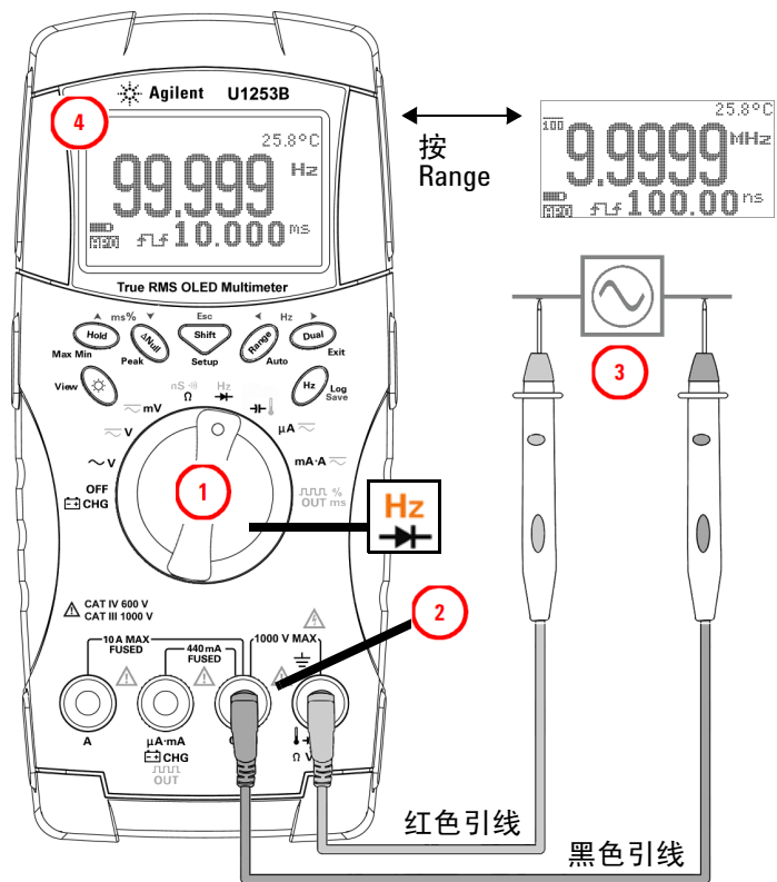
图 2-6 测量频率
