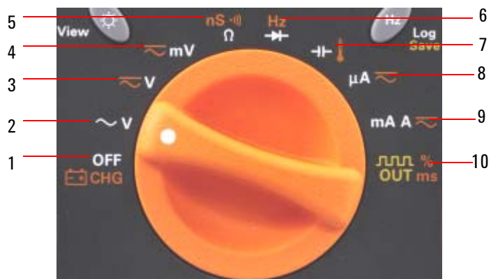
图 1-6 旋转开关
