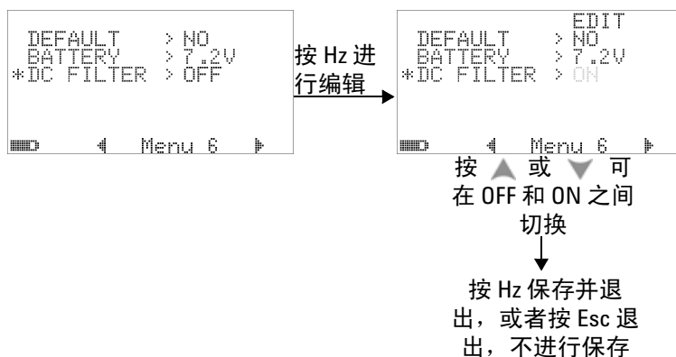
图 4-32 DC 滤波器
