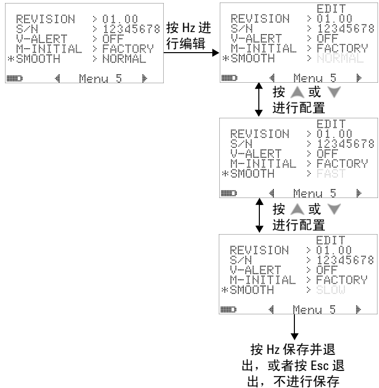
图 4-29 主显示屏读数的刷新率
