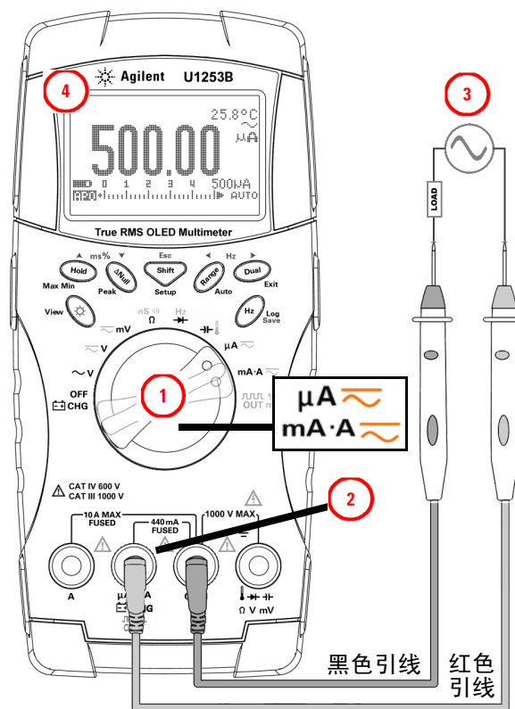
图 2-3 测量 \mu\text{A} 和 mA 电流
