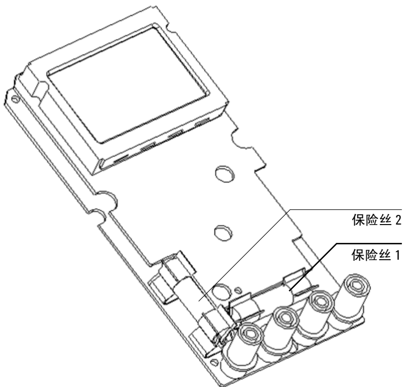
图 5-9 更换保险丝
