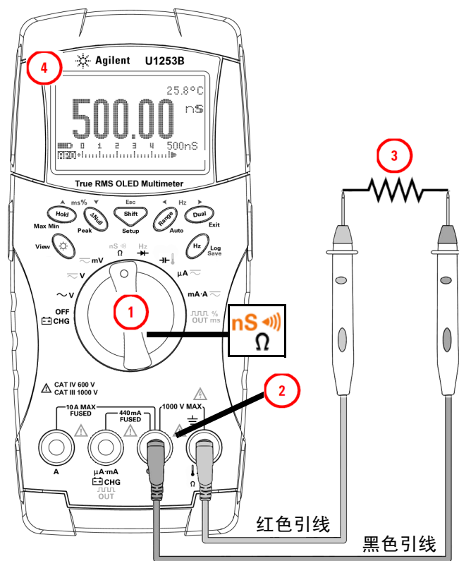
图 2-11 电导测量
