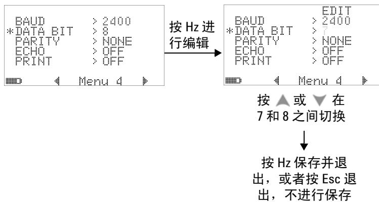
图 4-18 远程控制的数据位设置
