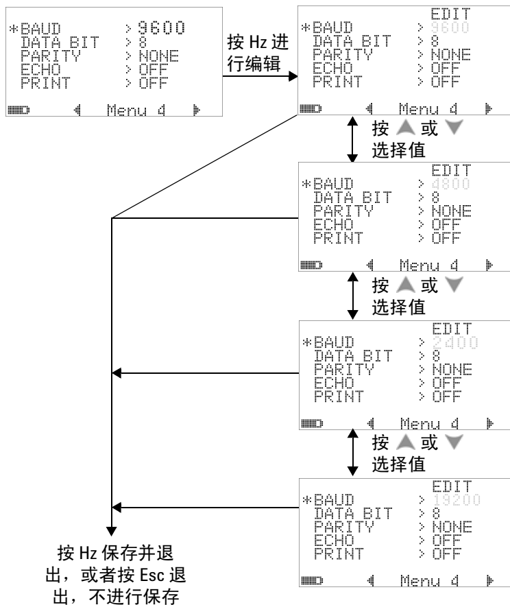
图 4-17 远程控制的波特率设置
