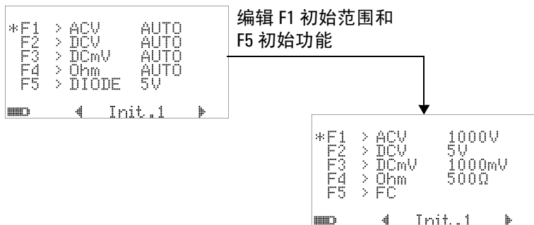
图 4-27 编辑初始测量功能 / 范围
