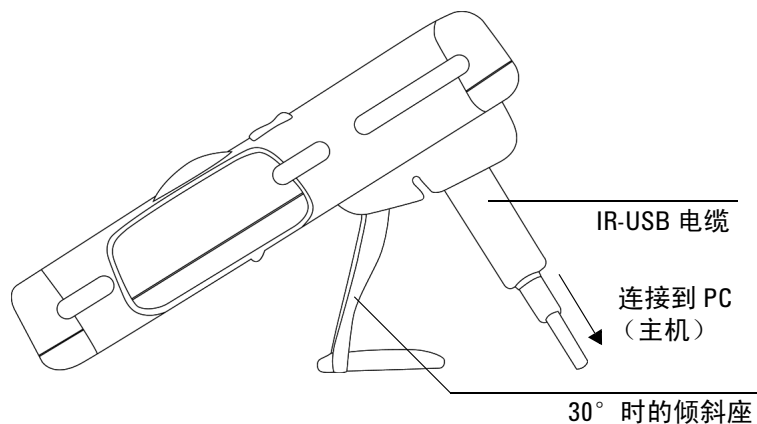
图 1-2 30° 时的倾斜座
