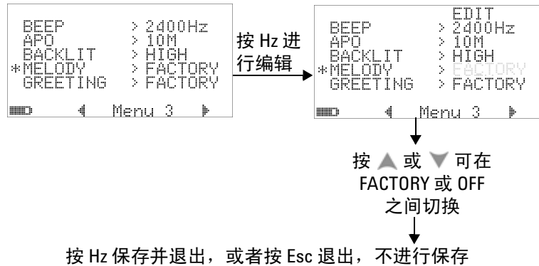
图 4-15 电源打开时的音乐设置
