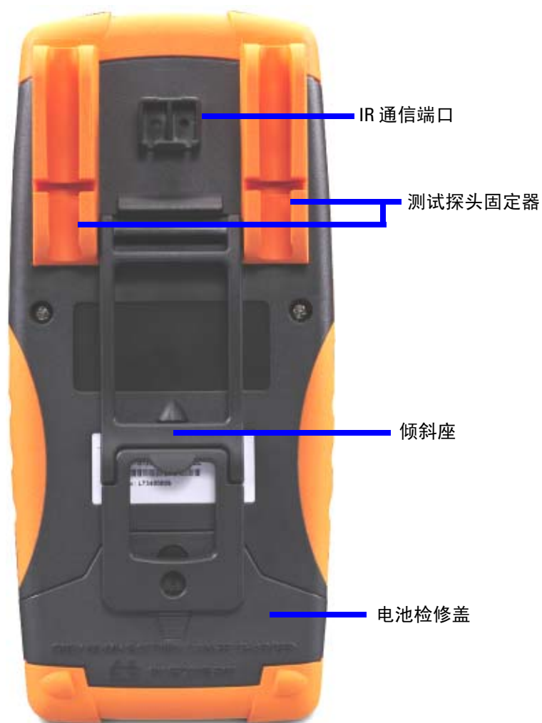
图 1-5 后面板
