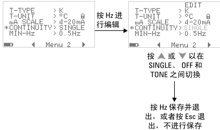
图 4-10 选择通断测试中所使用的声音
