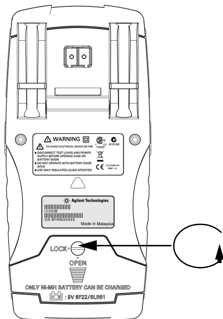
图 5-2 Agilent U1253B True RMS OLED 万用表后面板
