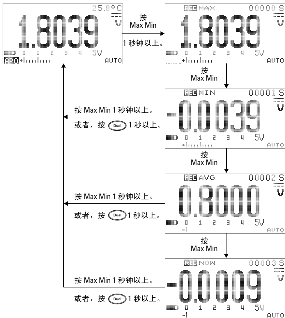
图 3-1 “Dynamic recording” 模式下的操作
