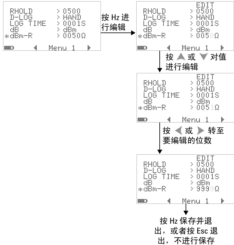
图 4-6 为 dBm 单位设置参考阻抗
