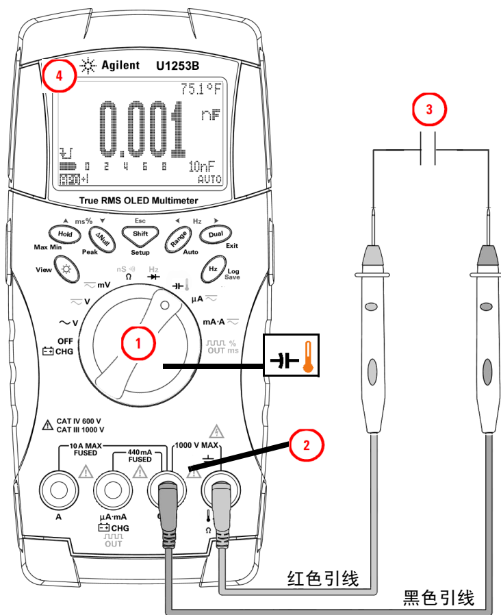
图 2-14 电容测量
