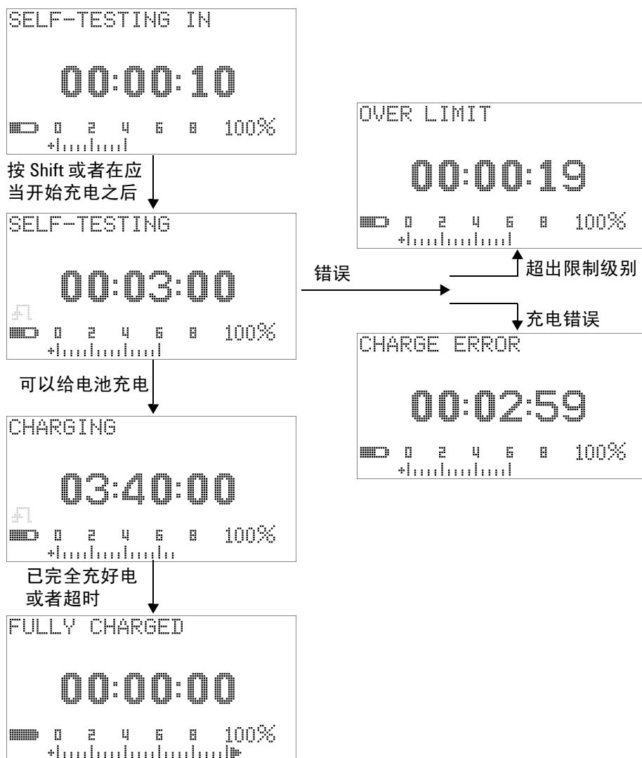
图 5-7 电池充电过程
