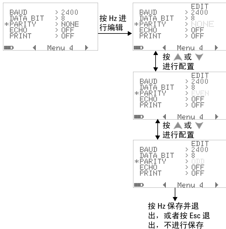
图 4-19 远程控制的奇偶校验设置
