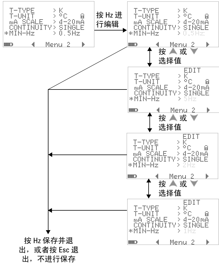
图 4-11 最小频率的设置
