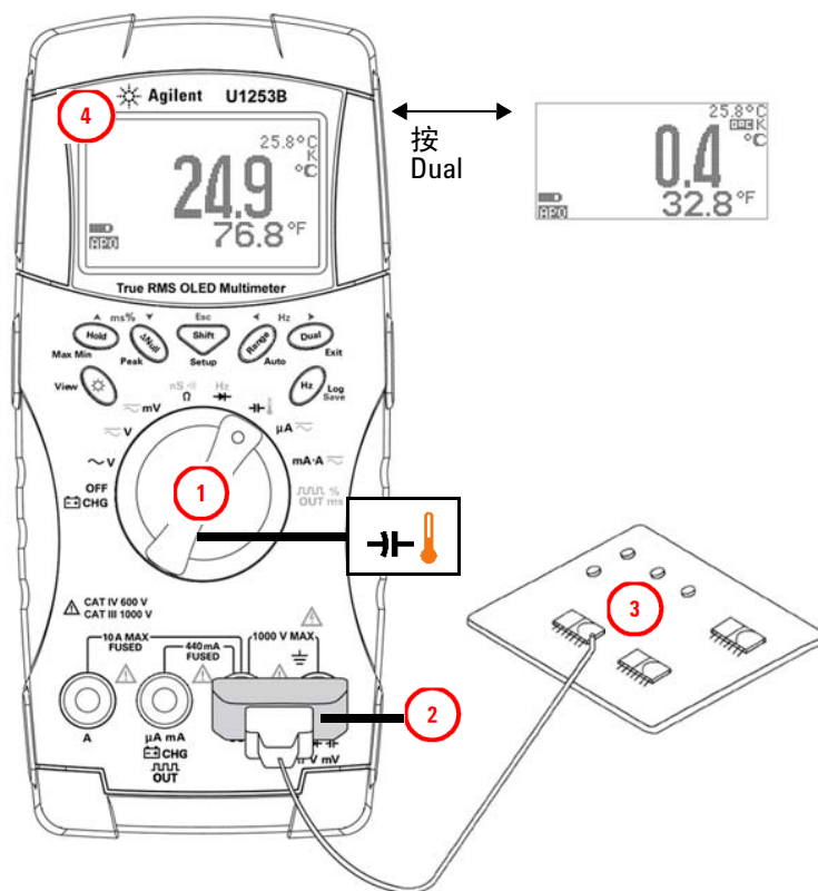
图 2-17 表面温度测量
