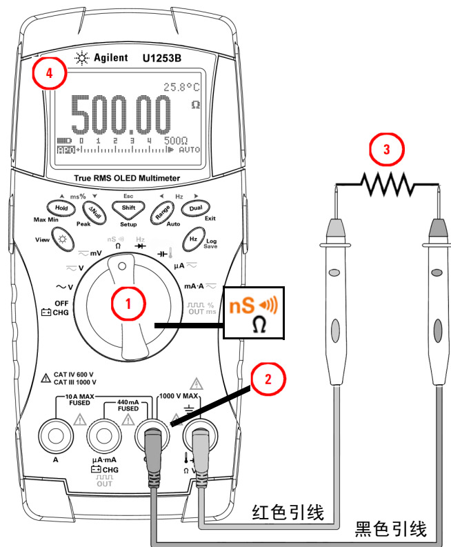
图 2-8 测量电阻
