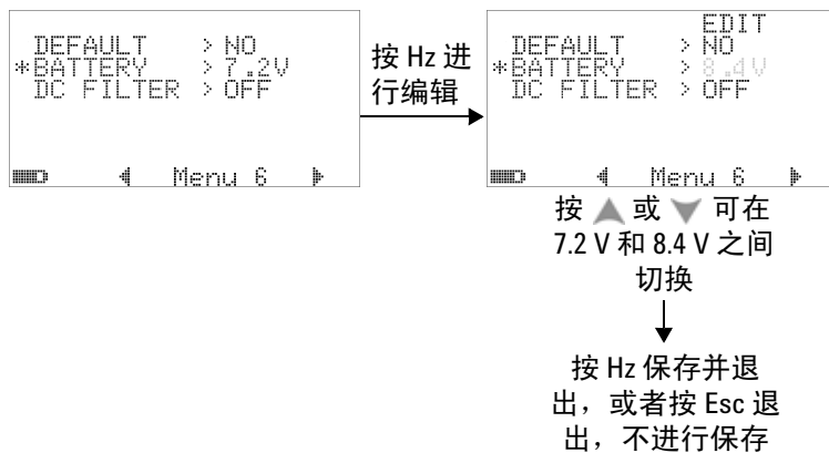
图 4-31 电池类型选择
