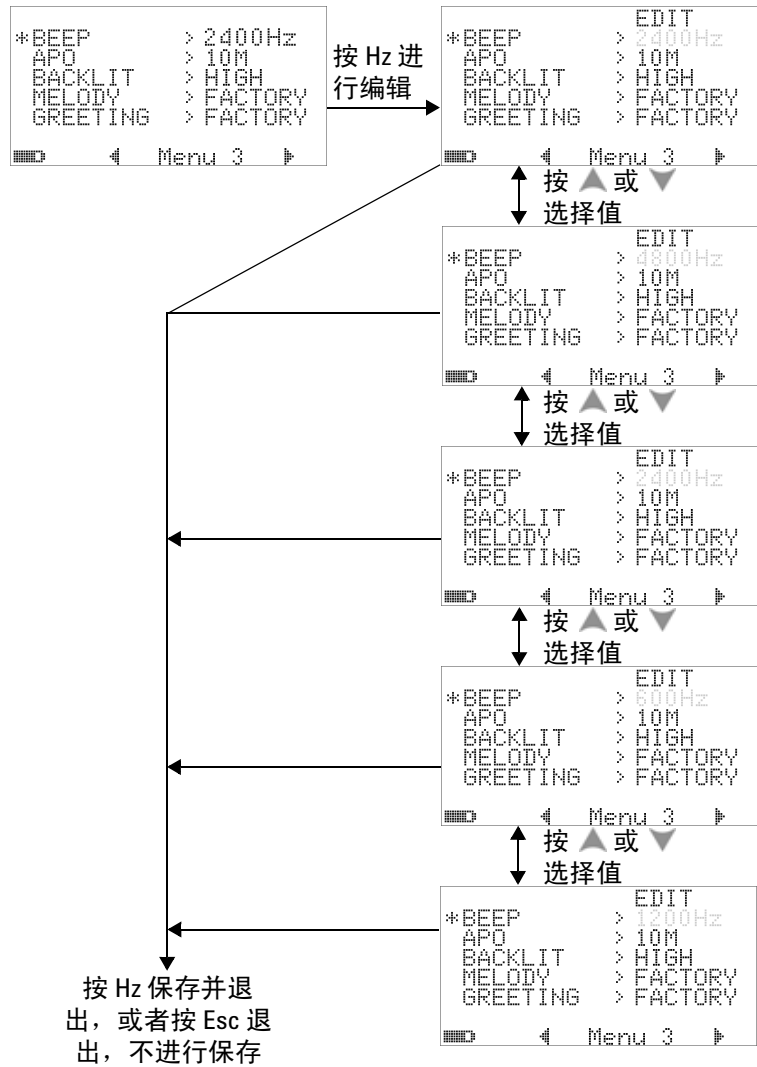
图 4-12 蜂鸣声频率的设置
