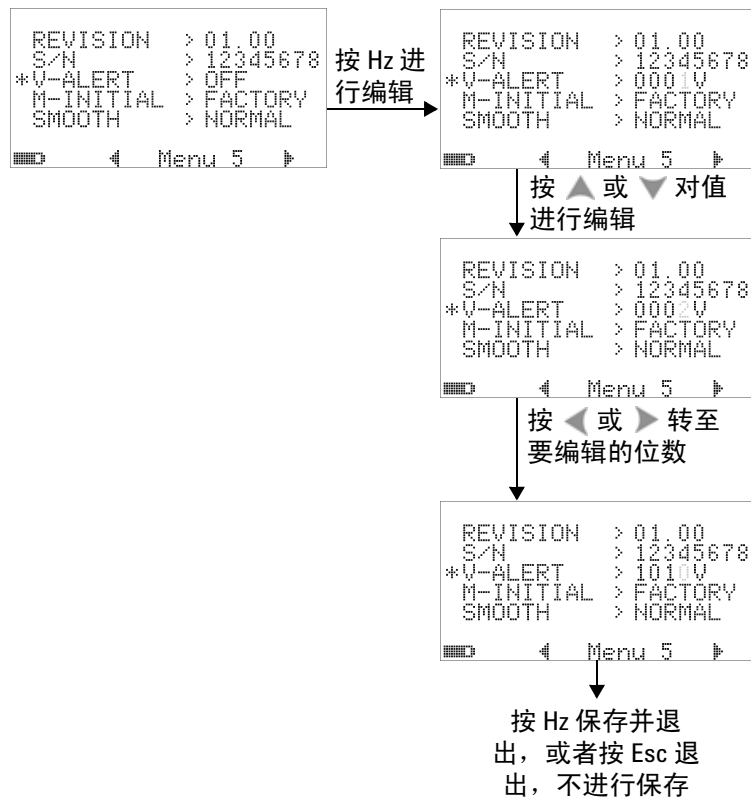
图 4-24 电压警报设置
